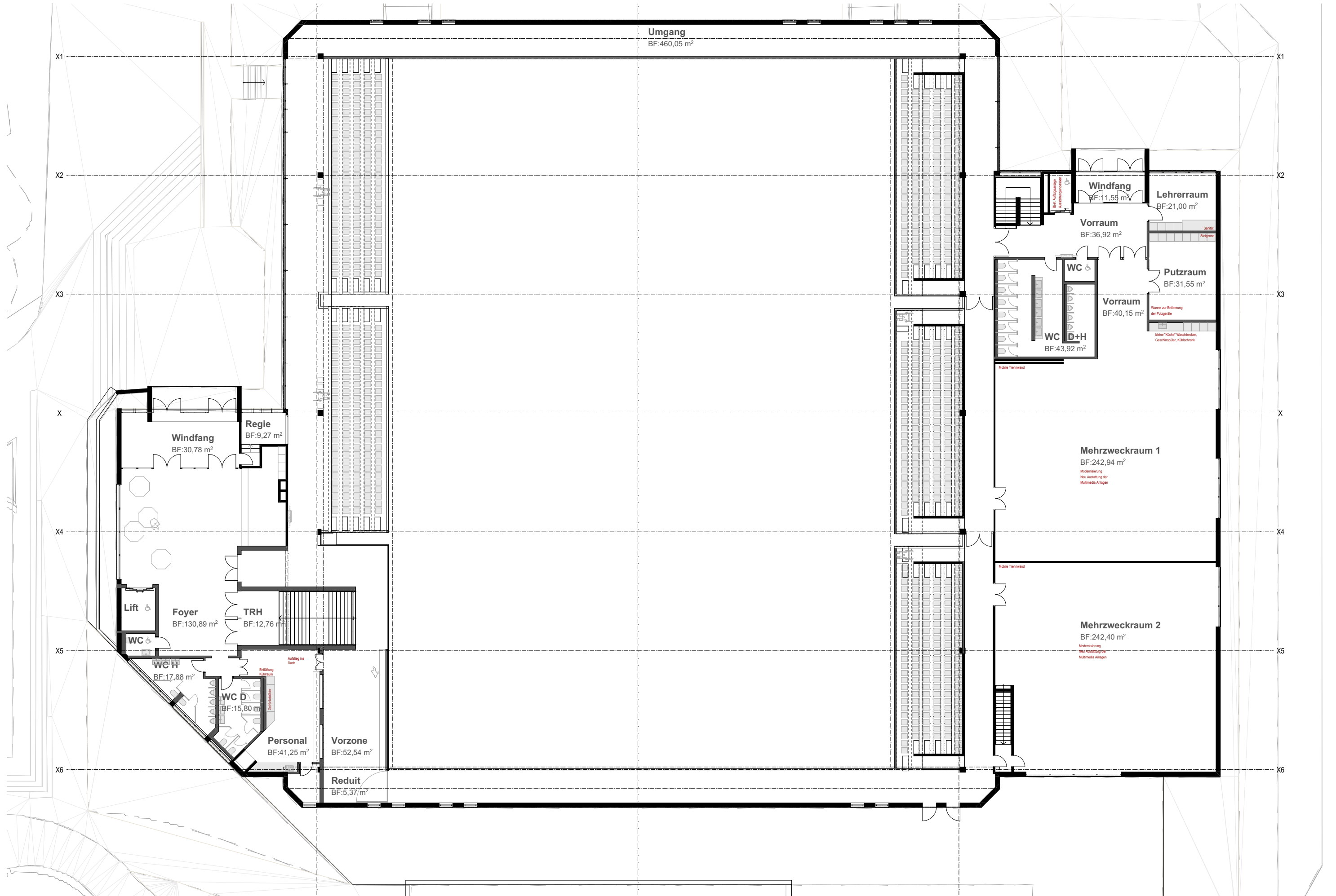
Eingangsniveau EG
